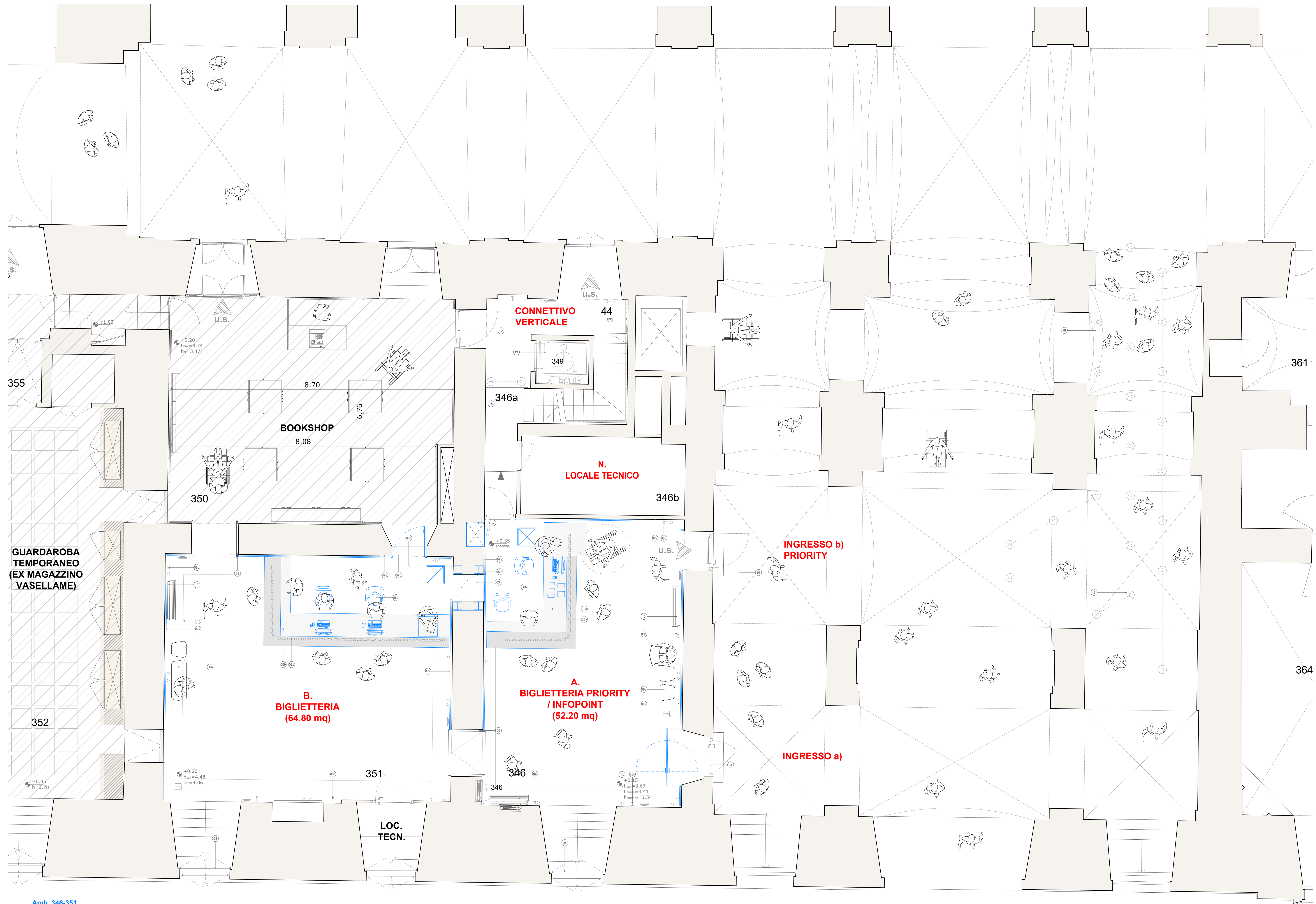
Amb. 346-351 PROGETTO Planimetria - scala 1:50
